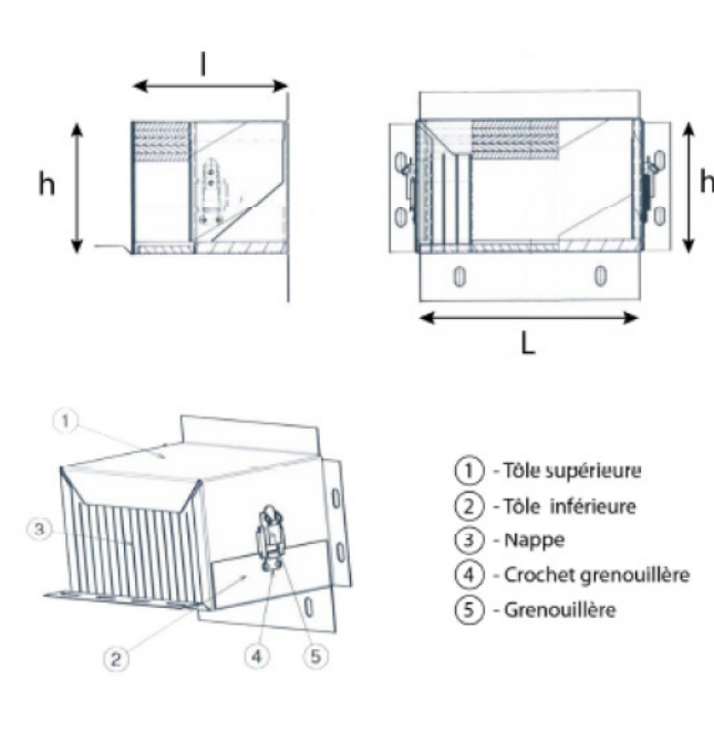
Schéma n°15 : Plan et dimensions boîtiers Gebsoboîtier coupe-feu
